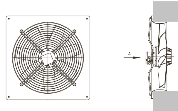
Rys. 1 . Montaż wentylatora wyciągowego WAF-S. Kierunek przepływu powietrza A.
